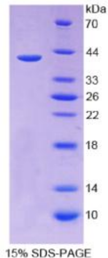
15% SDS-PAGE
