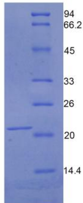
15% SDS-PAGE
